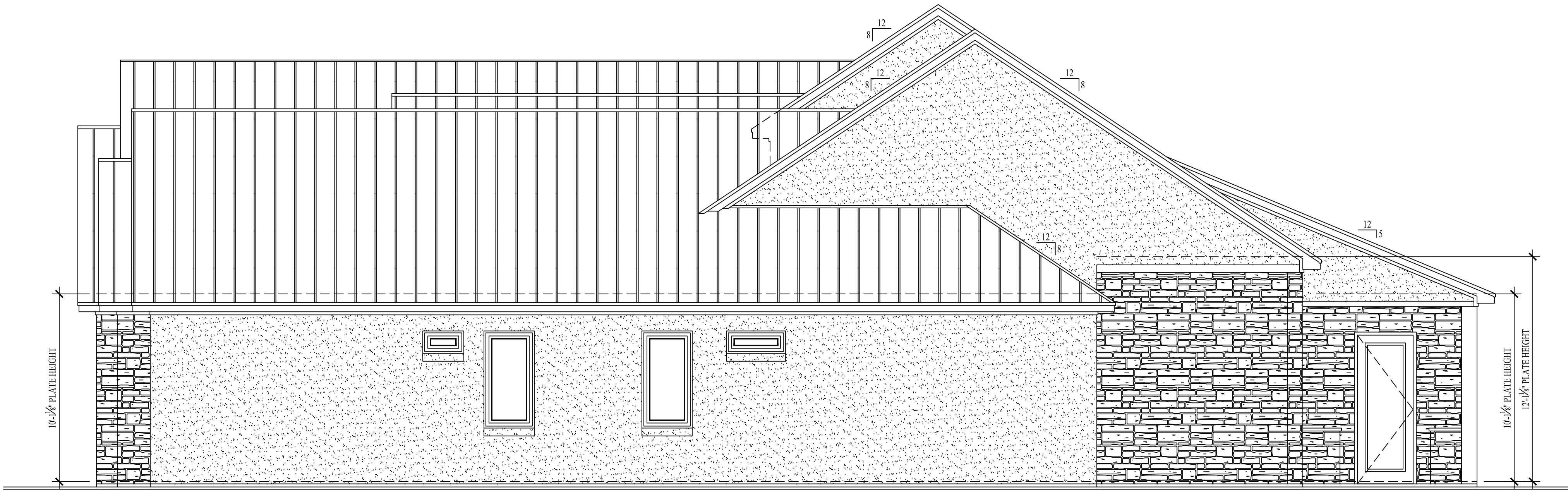
RIGHT ELEVATION
